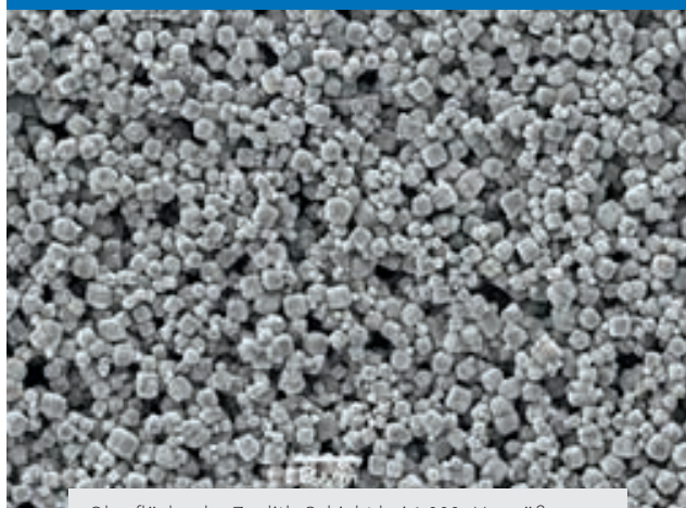
Oberfläche der Zeolith-Schicht bei 1 000x Vergrößerung.
